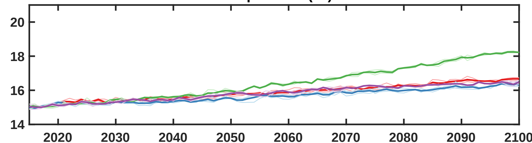
Global Surface Air Temperature (°C) - MPI-ESM1-2-HR
