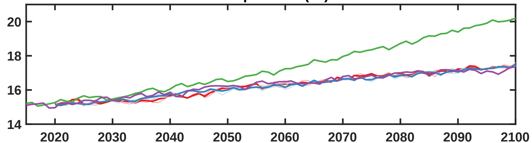
Global Surface Air Temperature (°C) - CESM2-WACCM
